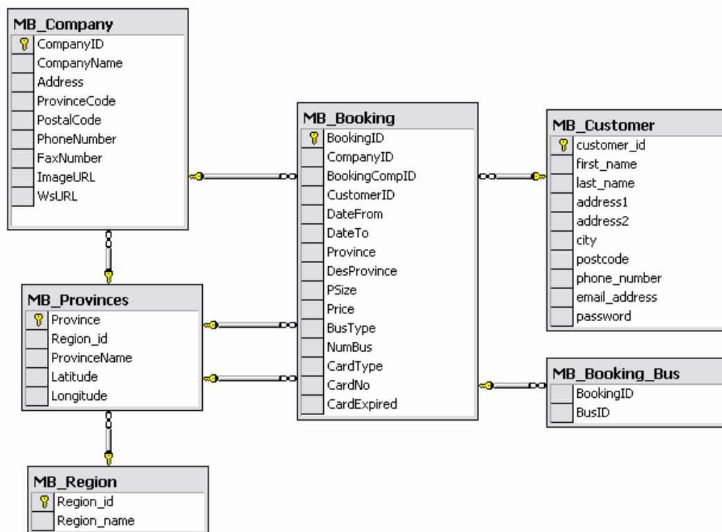
รูป 3.9 แสดง BusCenter Database Model Diagram
