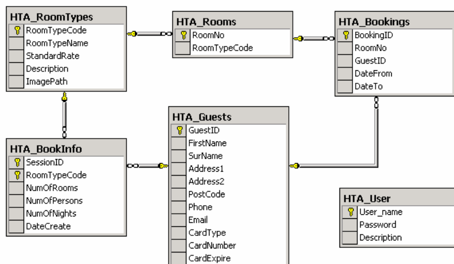
รูป 3.5 แสดง Hotel Database Model Diagram
