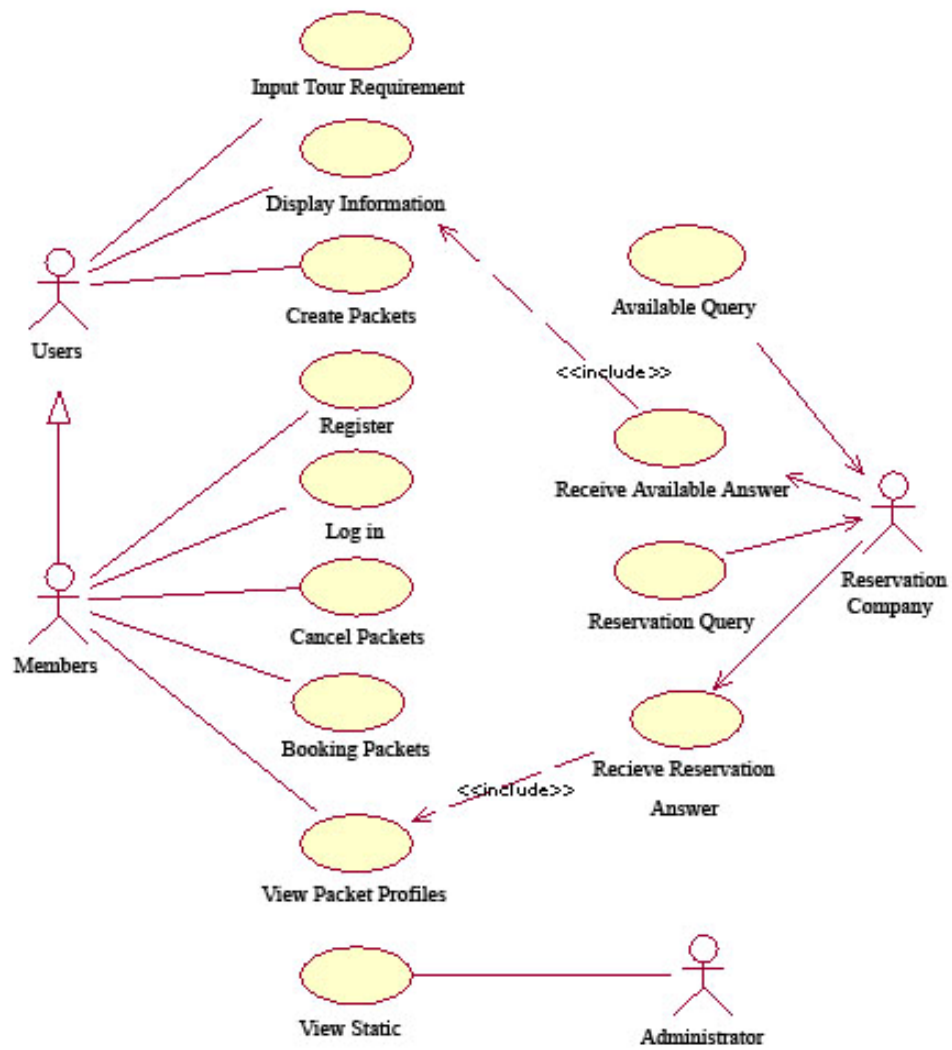
รูป 3.3 แสดง Use Case Diagram
