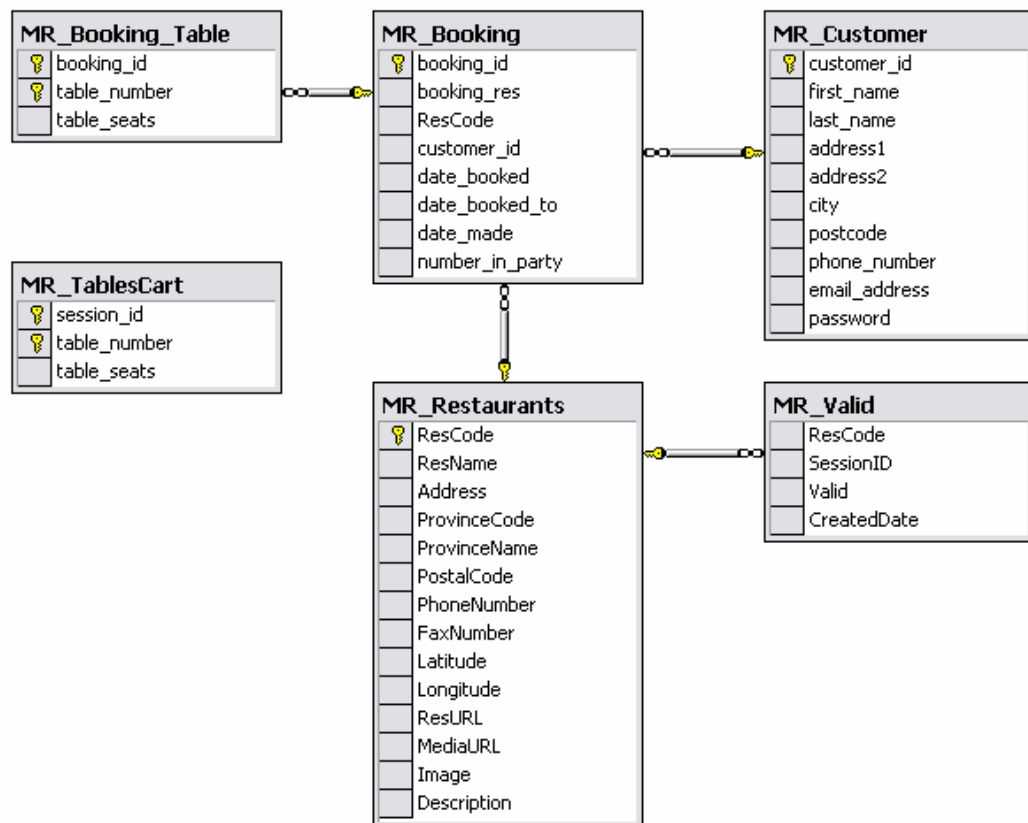
รูป 3.10 แสดง RestaurantCenter Database Model Diagram
